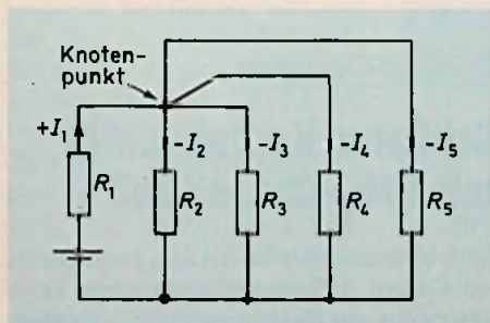
Bild 1. Bei der Stromverzweigung ist die Summe der zufließenden Ströme gleich der Summe der abfließenden
