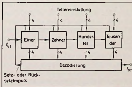
Bild 26. Auf- oder abwärts zählender programmierbarer Teiler. Ein fester Vorteiler liefert das Signal f_{VT}
